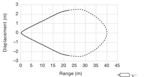
SMT 9x20 and SMR 9x20
